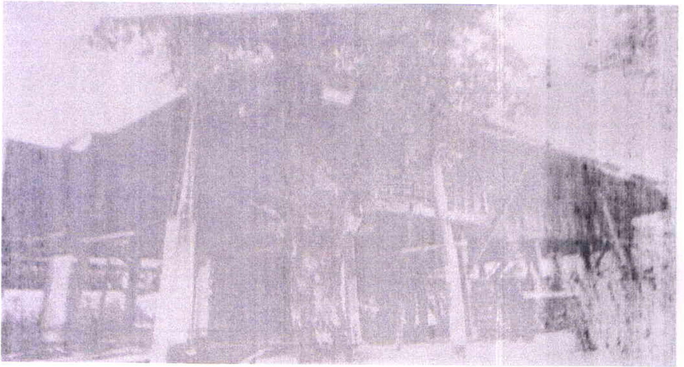
လွယ်တော်ခမ်းအုပ်စု၊ ကွင်းပြင်ဒေသ၊ ပါဝါးကျေးရွာ ၃၇'x၃၄'x၂၀'
